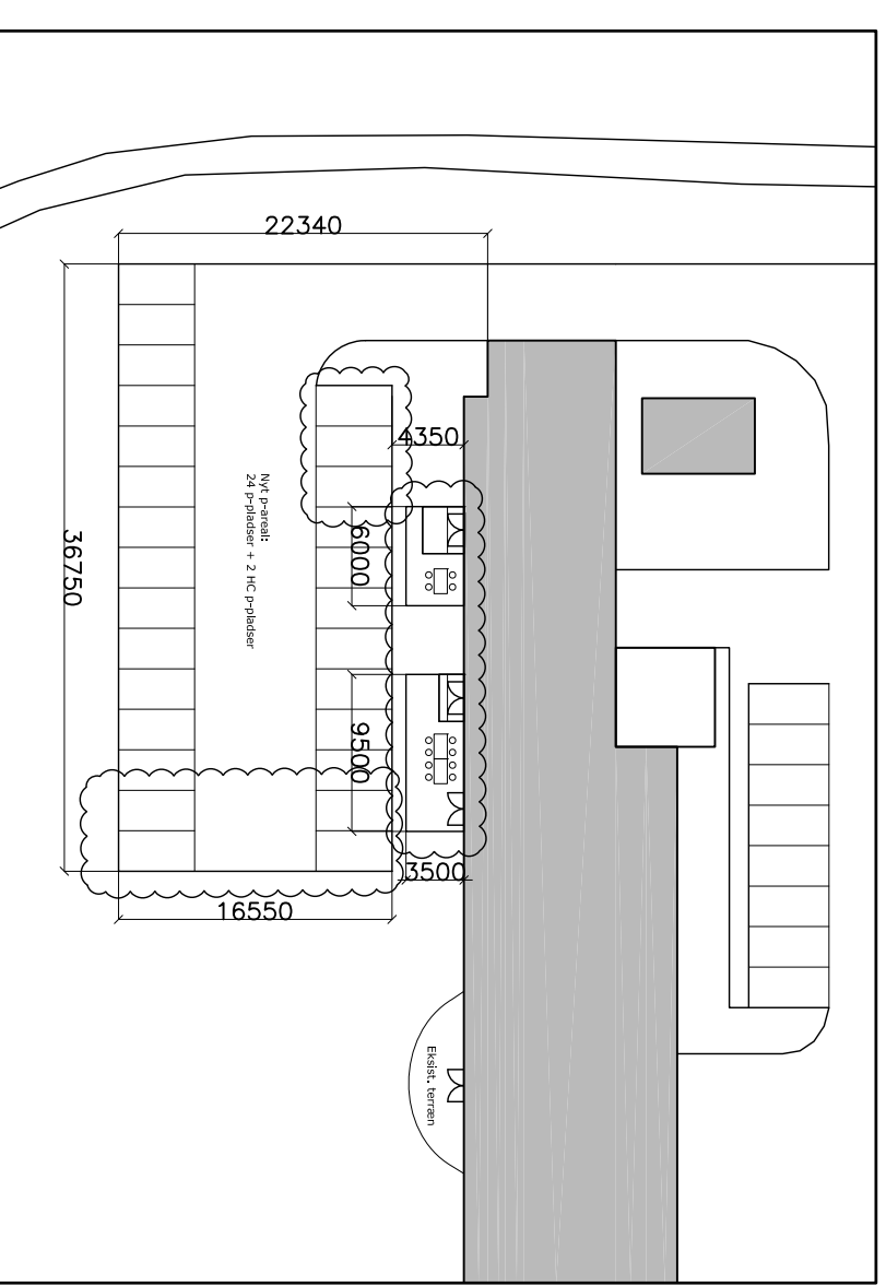
Udsnit af terræn - Nye forhold 1:500
