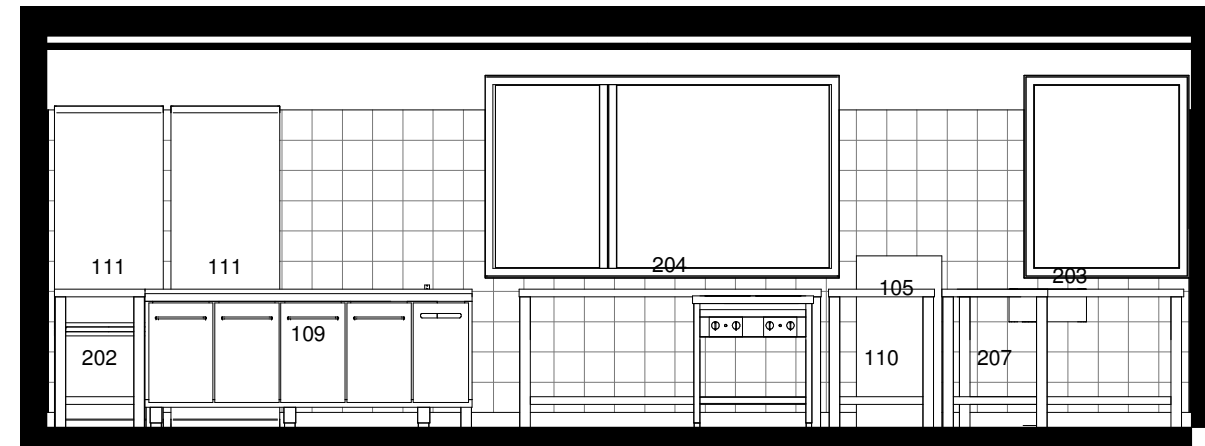
Opstalt B 1 : 50
