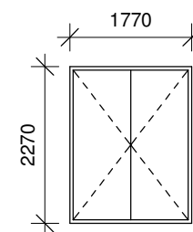
DA03 Udadgående dobbelt pladedør Inkl. sparkeplade Udføres som træ-/alu-parti
