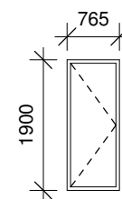
DA04 Udadgående pladedør Udføres som træ-/alu-parti
