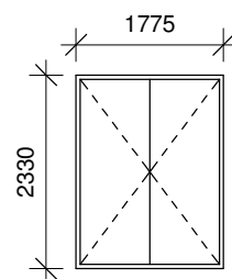
DA01 Udadgående dobbelt pladedør Inkl. sparkeplade Udføres som træ-/alu-parti
