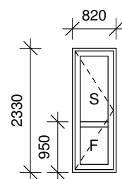
DA02 Udadgående facadedør Fyldning nederst, glas øverst Glas som cotswold glas Inkl. sparkeplade Udføres som træ-/alu-parti
