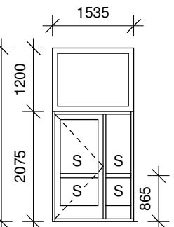
DH02 Udadgående dør med glas og sideparti samt glasparti med fast ramme over Udføres som træ-/alu-parti
