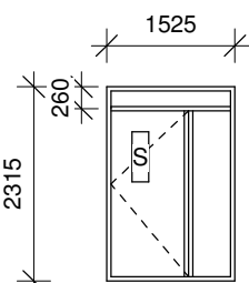
DH07 Indadgående pladedør med sideparti samt topparti med fyldning Mindre glasfelt i dør. Inkl. sparkeplade Udføres som træ-/alu-parti
