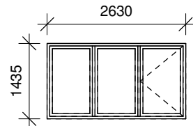
H17 Vinduesparti opdelt i tre felter ét felt udføres sidehængt med fluenet Udføres som træ-/alu-parti
