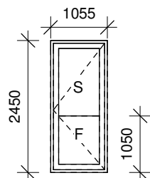
DH05 Udadgående dør Fyldning med glas øverst. inkl. sparkeplade Udføres som træ-/alu-parti *Vent. rist monteres på stedet
