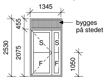
DH08 Udadgående facadedør Fyldning nederst, glas øverst Parti med vent. rist øverst. Inkl. sparkeplade Udføres som træ-/alu-parti
