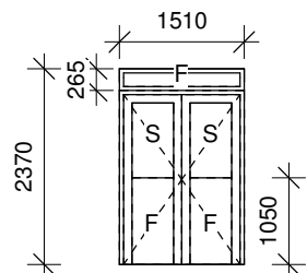
DH04 Indadgående dobbeltdør Med fyldning i bunden og glas i toppen. inkl. høj sparkeplade Fast felt med fyldning øverst Udføres som træ-/alu-parti
