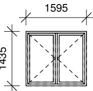
H16 Sidehængt vinduesparti Udføres som træ-/alu-parti
