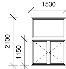
H13 Vinduesparti med sidehængt felt i bunden og glas med fast ramme i toppen. Et sidehængt felt udføres med fluenet. Udføres som træ-/alu-parti
