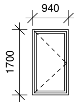
H09 Sidehængt vindue 3 venstre- og 2 højrehængslet Udføres som træ-/alu-parti
