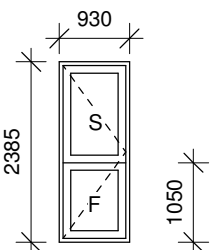
DH03 Udadgående facadedør Fyldning nederst, glas øverst Udføres som træ-/alu-parti
