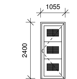
DH06 Indadgående facadedør Fyldninger med vent. riste. Inkl. sparkeplade Udføres som træ-/alu-parti *Vent. riste monteres på stedet
