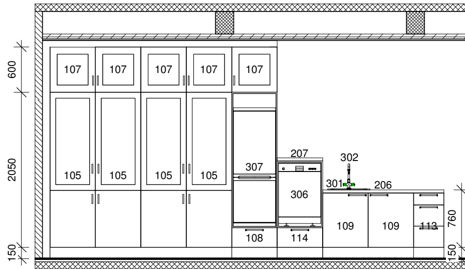
S11 - A 1 : 50
