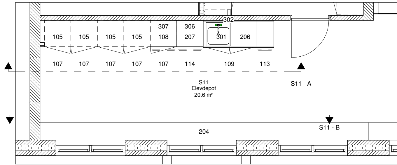
Stuen - S11 1 : 50
