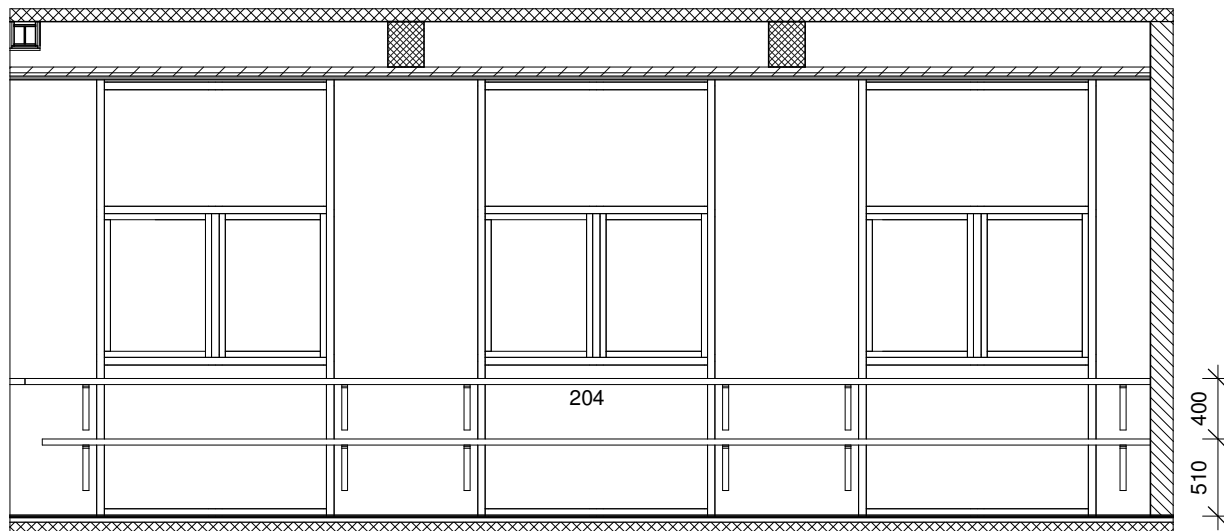
S11 - B 1 : 50
