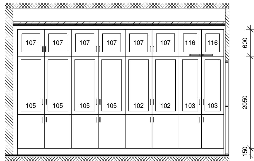
S10A - B 1 : 50
