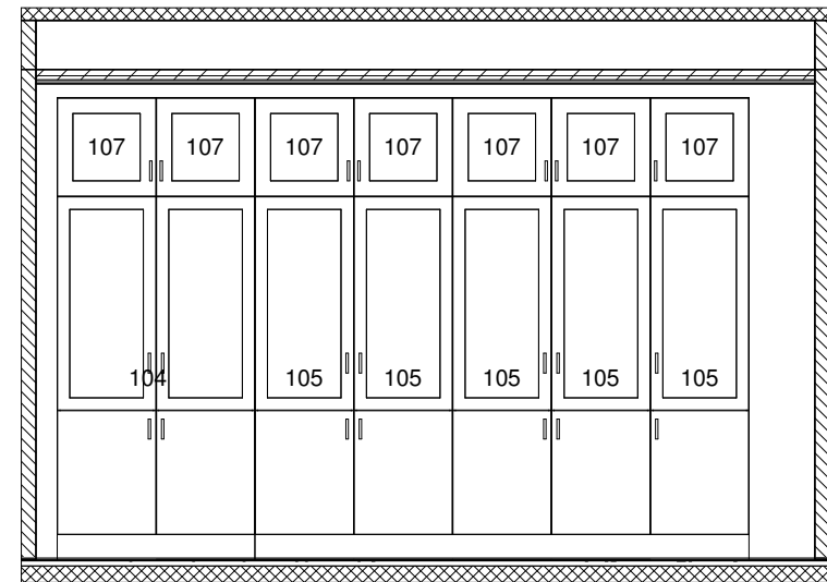
S10A - A 1 : 50
