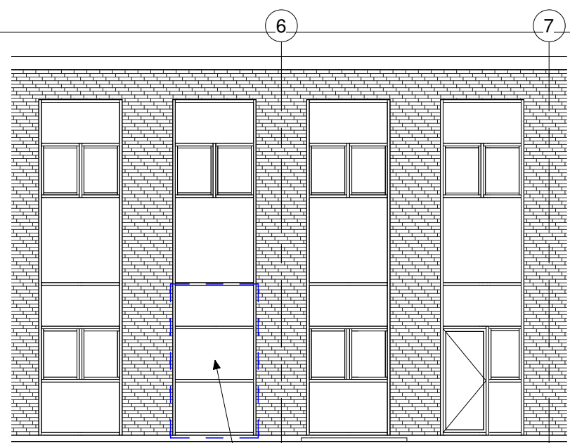
Facadeudsnit 1 : 100
