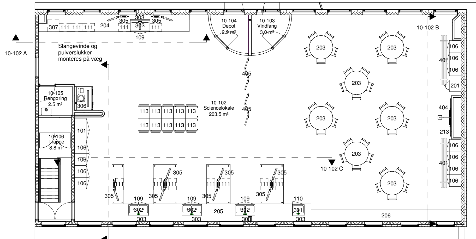
Rumtegning 10-102 10-102 D 1 : 100
