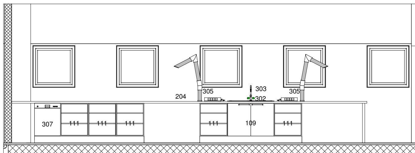
10-102 A 1 : 50
