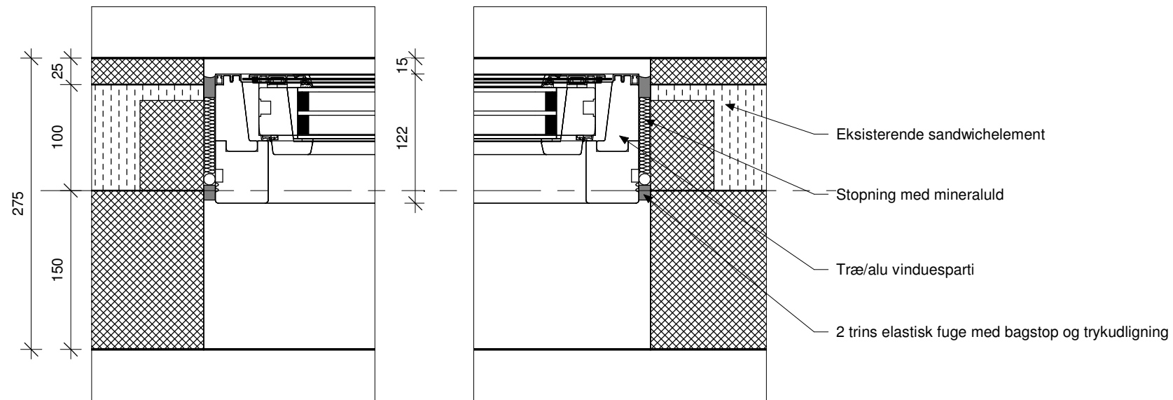
Vandret detalje - vindue
