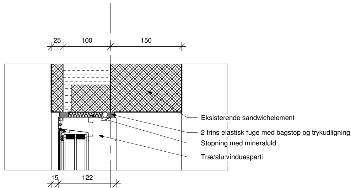
Vandret detalje - vindue
