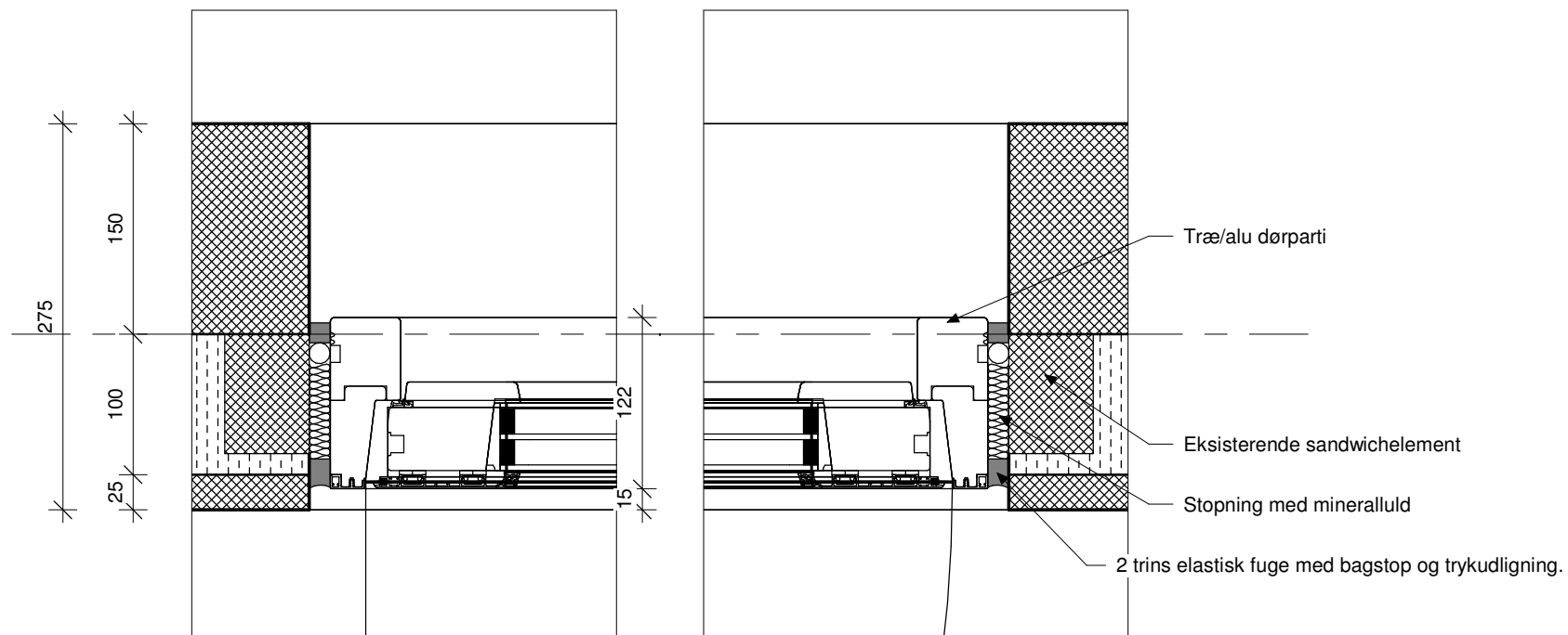
Vandret detalje - dør
